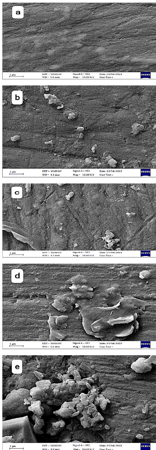
Figure 6. FESEM images: (a) pure Al; (b) Al + 0.5 ZnO + 0.5 Gr; (c) Al + 1.5 ZnO + 0.5 Gr; (d) Al + 2.5 ZnO + 0.5 Gr; (e) Al + 3.5 ZnO + 0.5 Gr.
